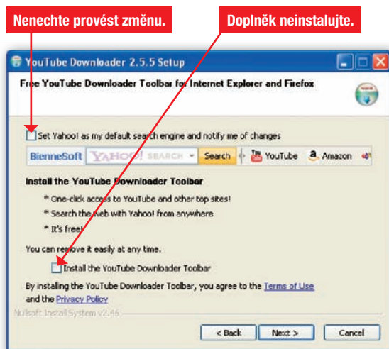
OBR. 2 Instalace programu.
